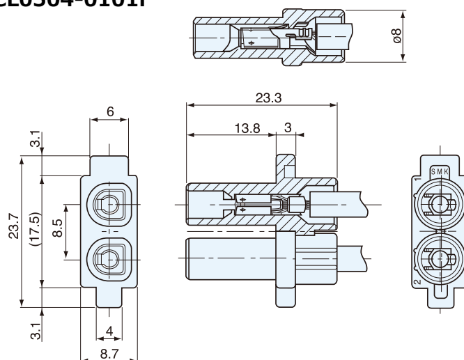
Socket : CCL0504-0101F
