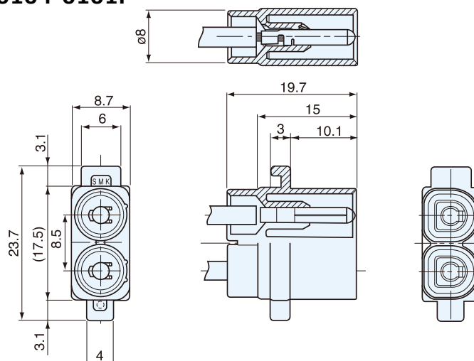
Plug : CCT0104-0101F
