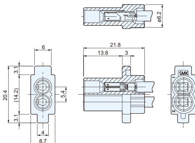
Socket : CCL0505-0100F
