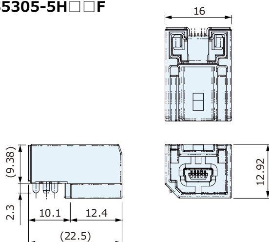
Socket : CSS5305-5H□□F
